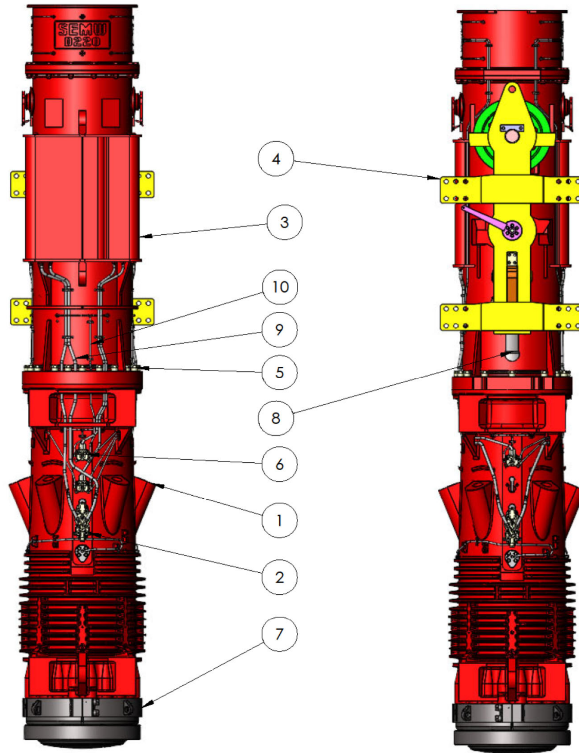
D220 HAMMER P#: 195.00
