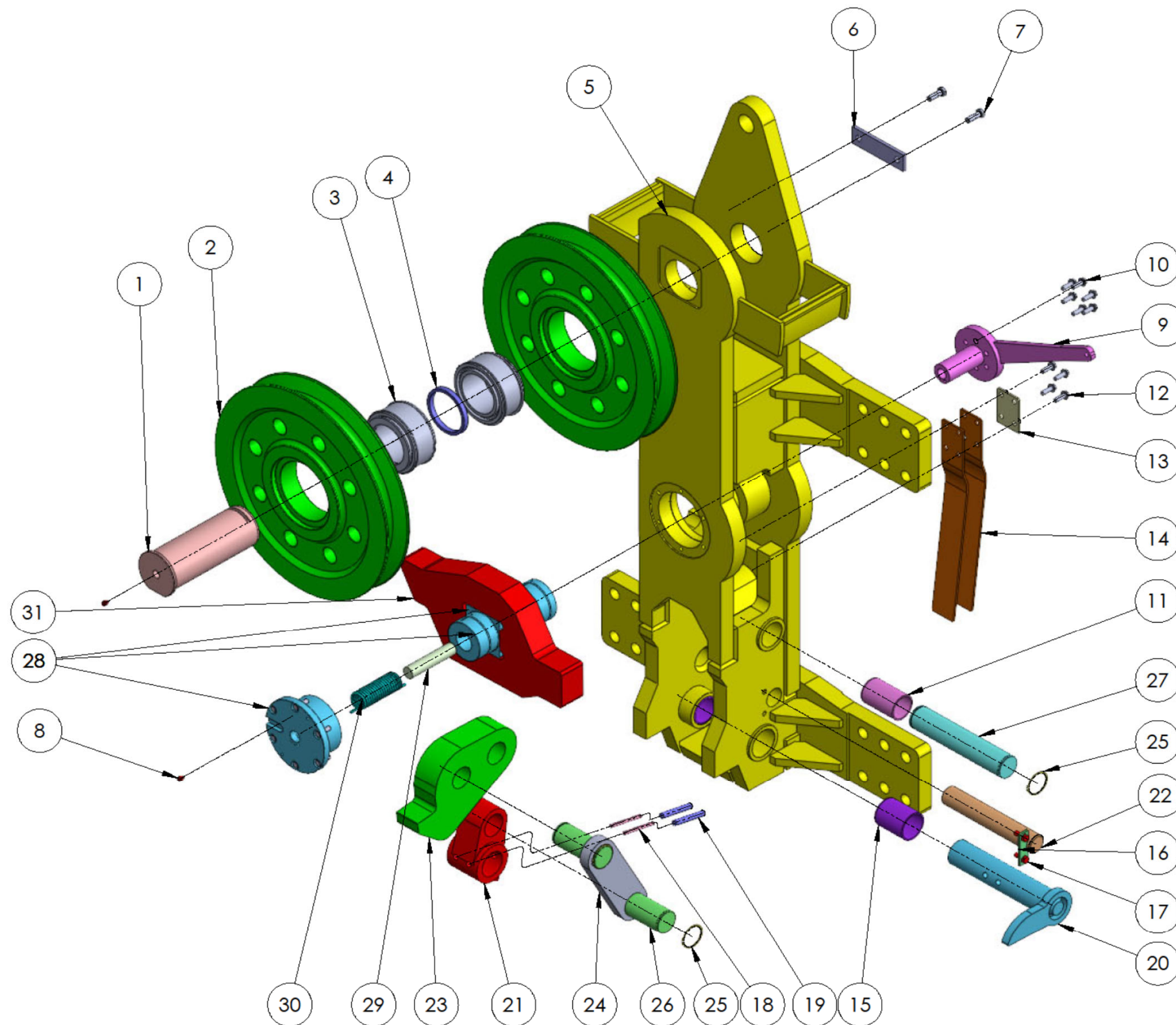
TRIP SLED CPL(D220) P#: 195.05.00
